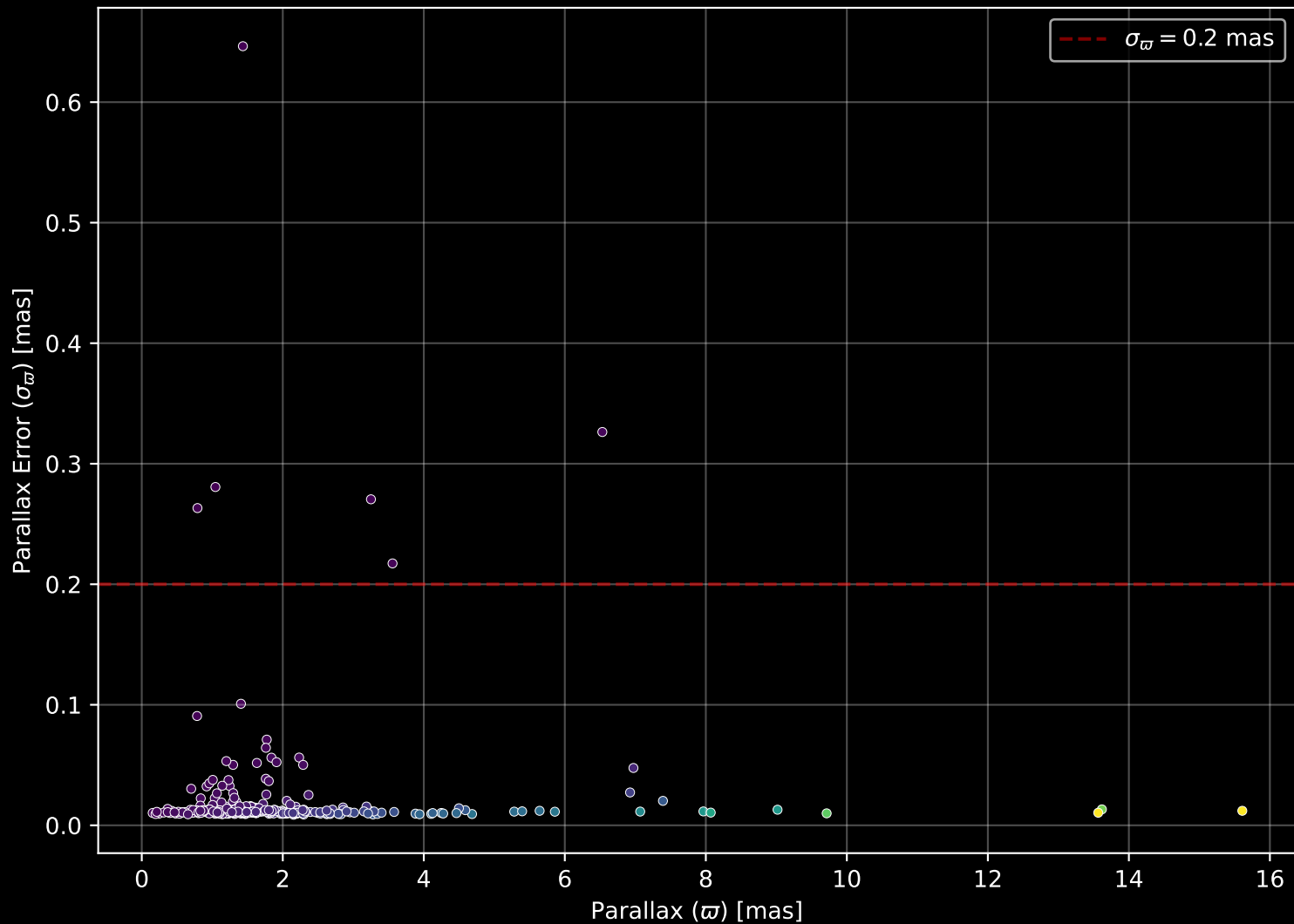
GALAH DR4 Field: [557] Parallax Quality (n= 306)
