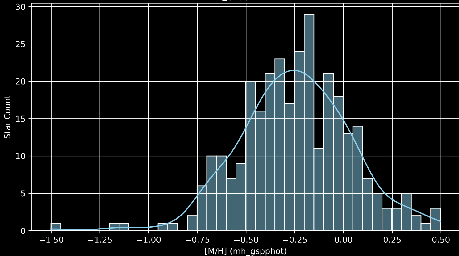
GALAH DR4 Field: [557] [M/H] (mh_gspphot) (n= 305)
