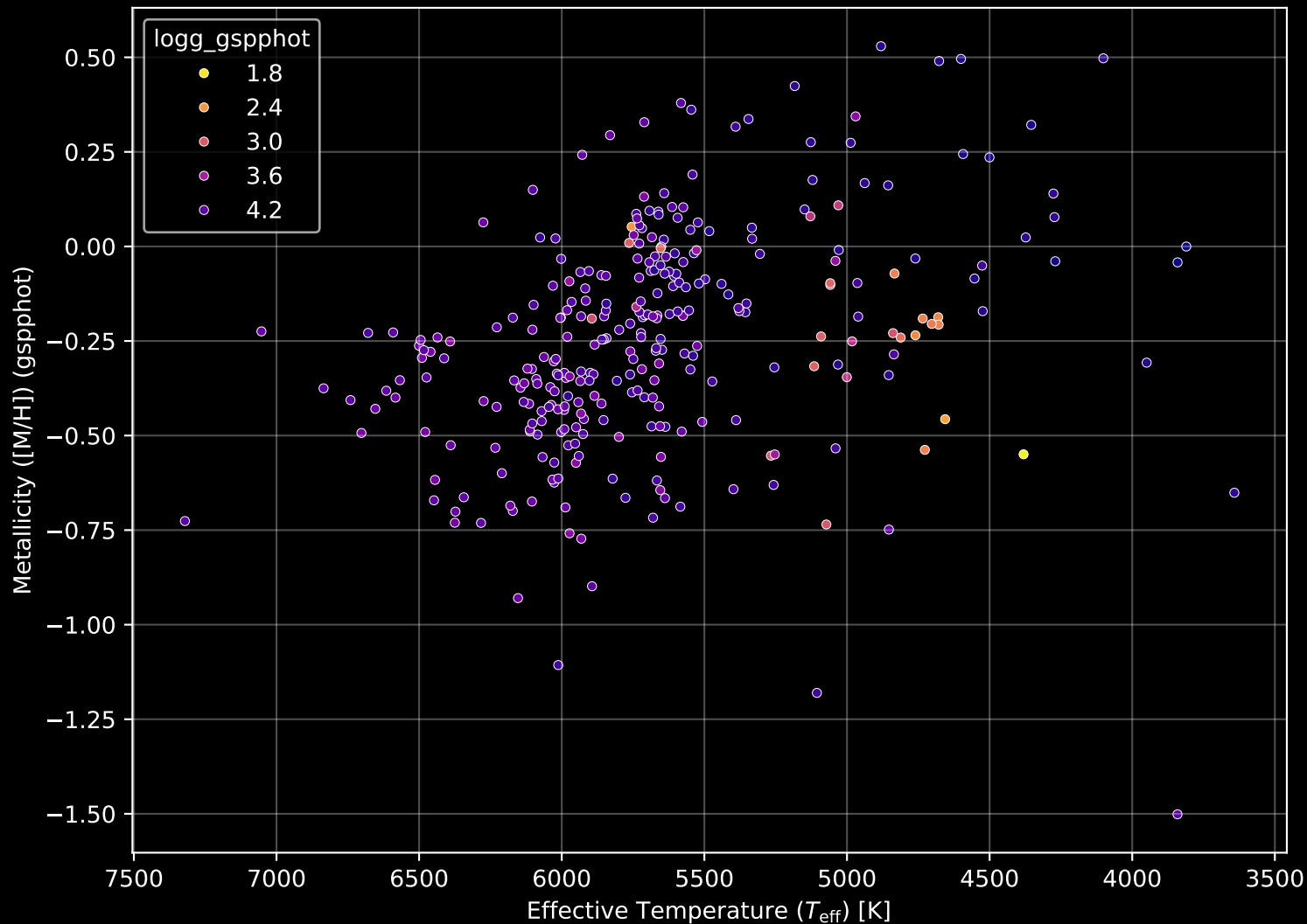
GALAH DR4 Field: [557] Stellar Population Parameters (n= 306)
